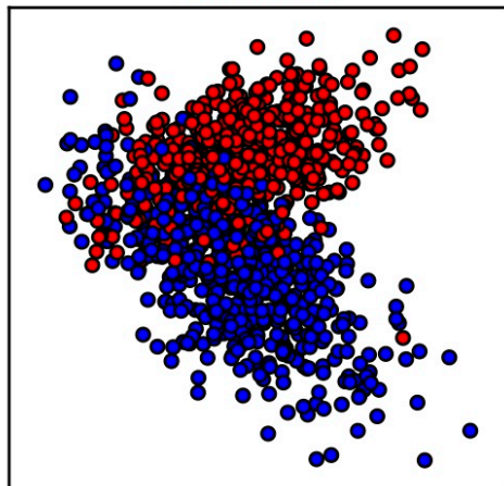
Dataset
